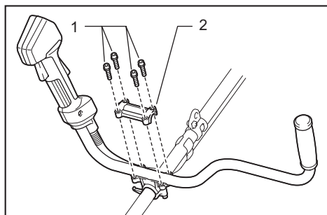
► 1. Boulon à tête creuse hexagonale 2. Serre-guidon
