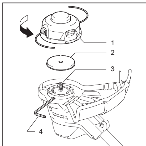
► 1. Cabezal de corte de nylon 2. Protector metálico 3. Eje 4. Llave hexagonal
