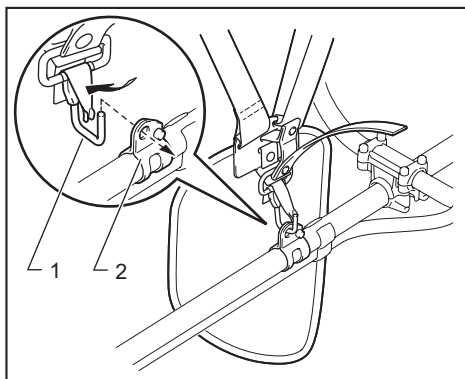
► 1. Hook 2. Hanger
