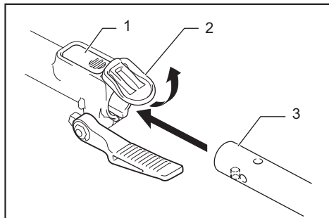
► 1. Palanca de bloqueo 2. Cubierta de la junta 3. Tubo
