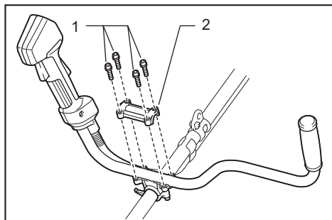
► 1. Perno de cabeza hueca hexagonal 2. Abrazadera del mango
